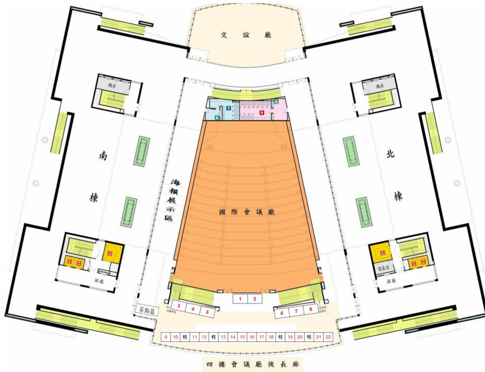
國際會議廳 4F 平面圖
